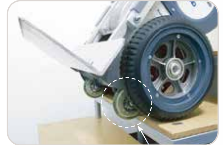
계단 끝 감지 휠
